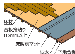
【床暖フローリング施工時】
