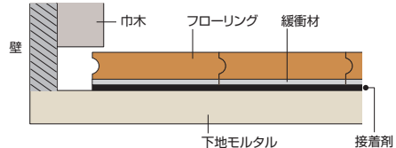
直貼り工法(モルタル下地)
