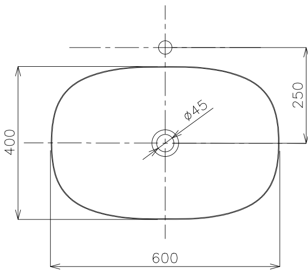
平面図
