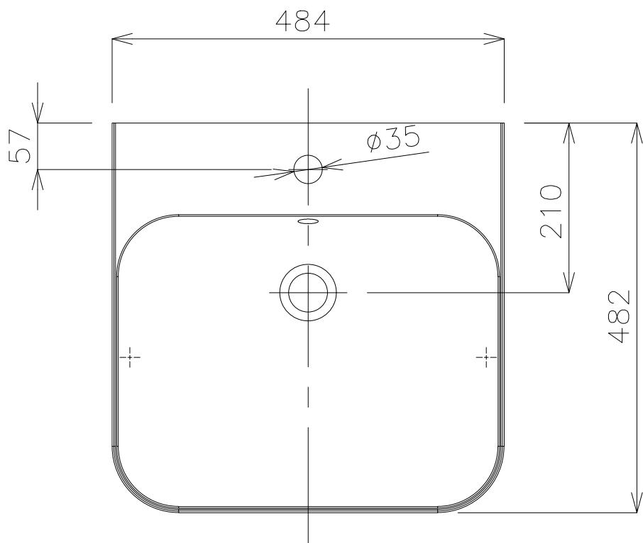
平面図
